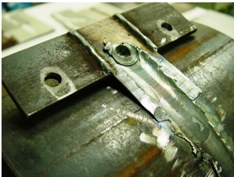
Figura 3: Lingüeta para escape posicionada no final da soldagem circunferencial de tubo [Feng 2005].
