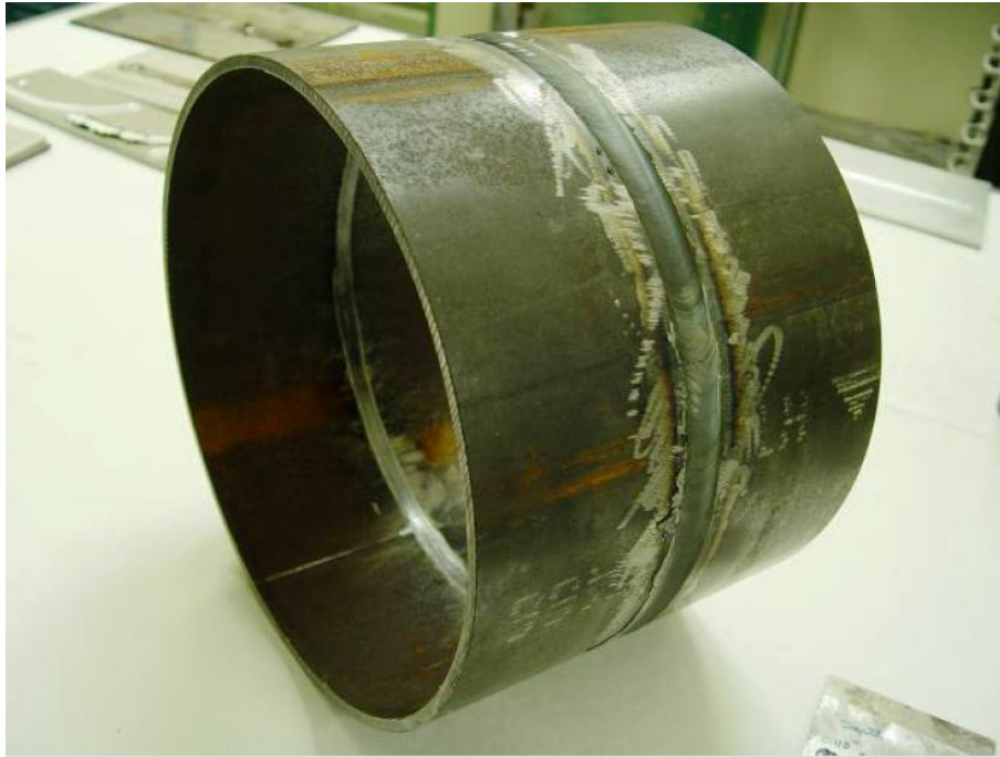
Figura 7: Aspecto final do cordão de soldagem circunferencial feito através do processo de fricção linear em tubo grau API X65 [Feng 2005].
