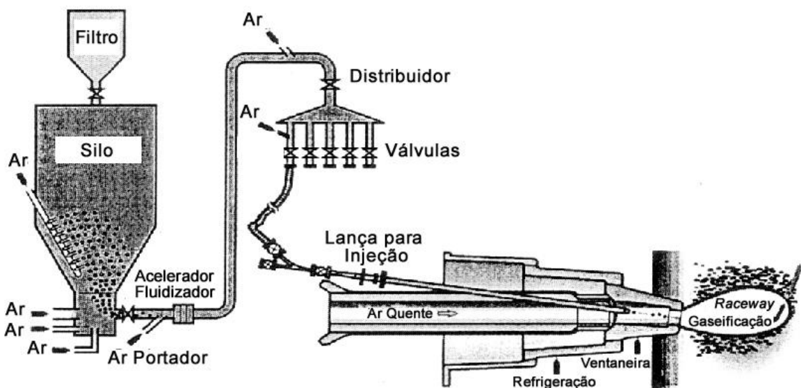
Figura 6: Esquema de injeção da mistura de ar mais grânulos de sucata plástica no alto-forno [WAKITA 2002].
