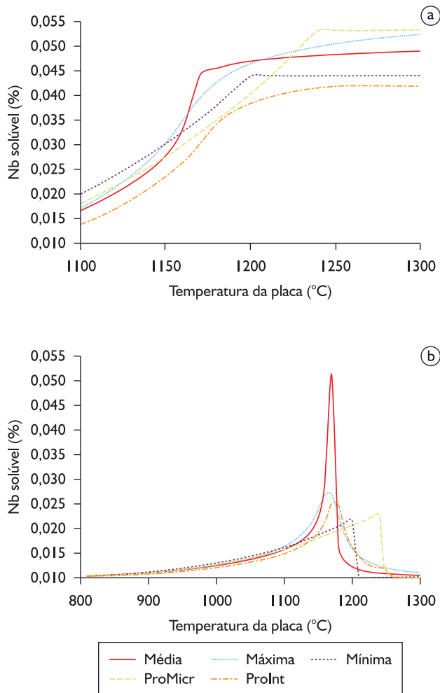
Figura 2. a) Evolução do teor de Nb solubilizado ao longo da temperatura e b) taxa de sua solubilização em relação à temperatura para as ligas mostradas na Tabela 1.
