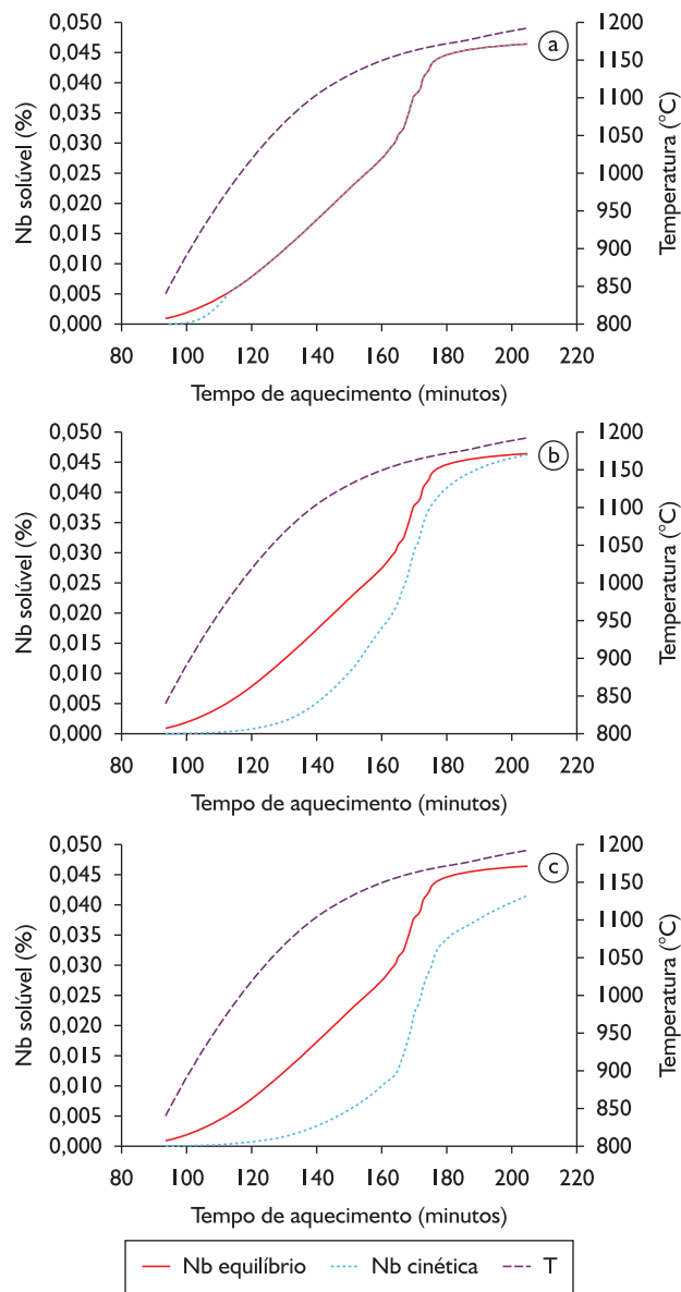
Figura 1. Evolução da solubilização prevista do Nb e da temperatura no interior da placa ao longo do tempo de reaquecimento para o aço aqui estudado. Tamanho de precipitado: a) 17 nm; b) 250 nm; e c) 500 nm.
